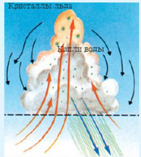
Рис. 3: Кучево-дождевое облако. После того как облако вырастает в высоту, начинается дождь. (Weather and Climate [“Погода и климат “], Бодин (Bodin), стр .123.)
