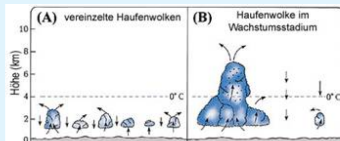
Abbildung 2: (A) Einzelne kleine Wolkenstücke (Cumuluswolken). (B) Wenn kleine Wolken sich vereinigen, lassen Aufwinde die größere Wolke anwachsen, bis die Wolke aufgeschichtet ist. Wassertropfen werden durch □ Punkte gekennzeichnet. ( The Atmosphere [Die Atmosphäre], Anthes und andere, S.269.)
