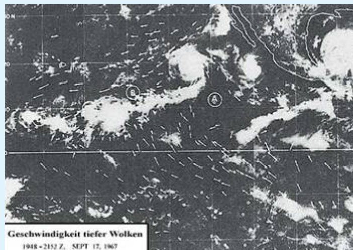
Abbildung 1: Satellitenaufnahmen zeigen wie sich die Wolken zu den Konvergenzzonen B, C und D bewegen. Die Pfeile zeigen die Windrichtungen an. ( The Use of Satellite Pictures in Weather )
